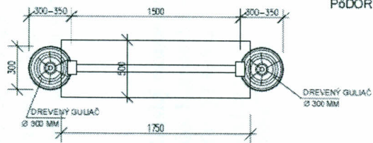
Pôdorys
