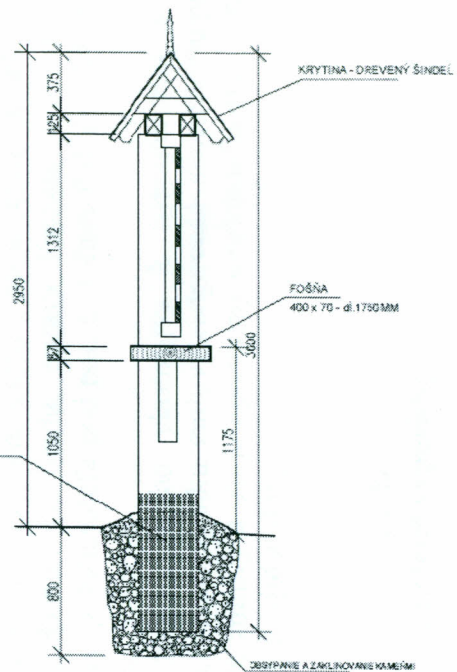
ZVISLÝ REZ
